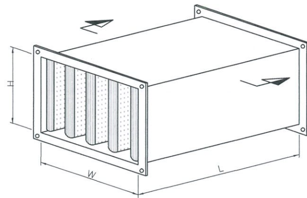
소음기 상세도
