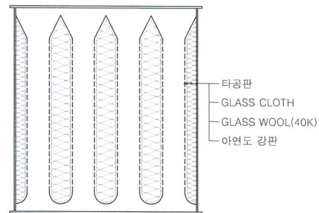
단면상세도
