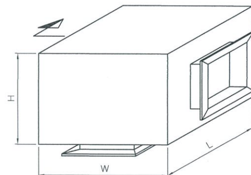
소음챔바상세도
