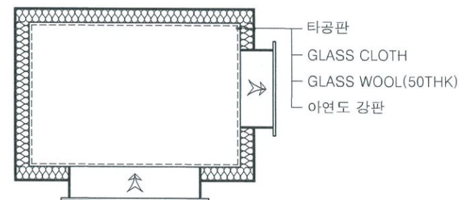
단면상세도
